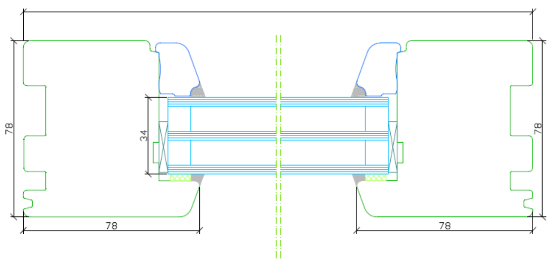
Horizontal crosscut width
